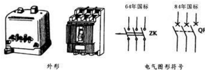
图5-9 空气断路器
