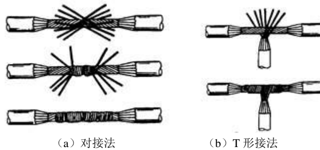
图 1-17 多股导线接法
