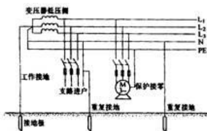
图 3-1 工作接地、重复接地
