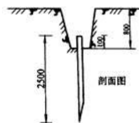
图 3-3 垂直接地体
