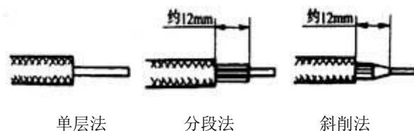
图 1-15 电线头的削法
