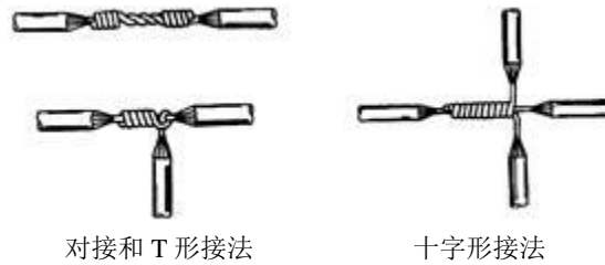
图 1-16 单股导线接法
