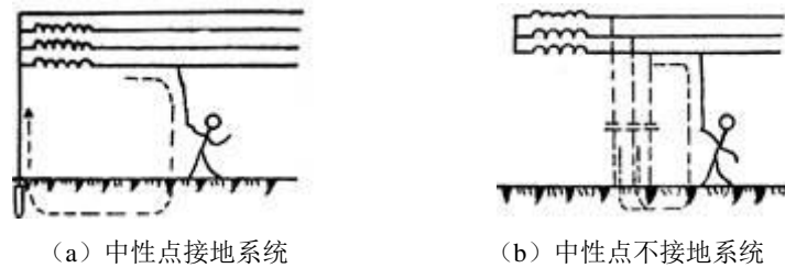
图 2-1 单线触电
