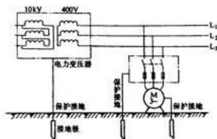
图 3-2 保护接地
