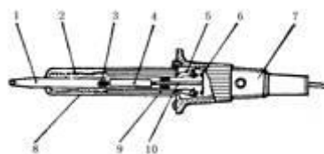
图 1-8 电烙铁
