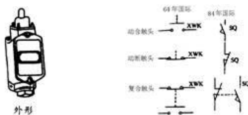
图 5-8 行程开关
