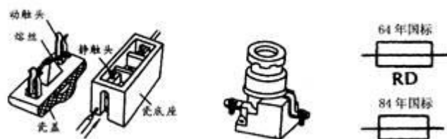
图 5-4 熔断器
