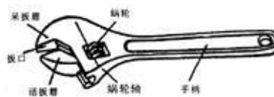
图 1-6 活扳手
